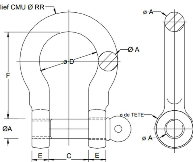
Forme Lyre Suivant norme 83 302
