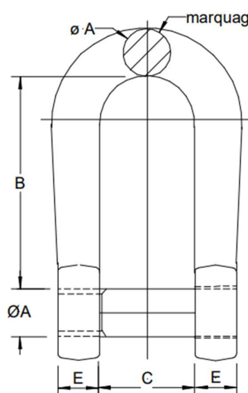
Forme Droite Suivant norme 83 301
